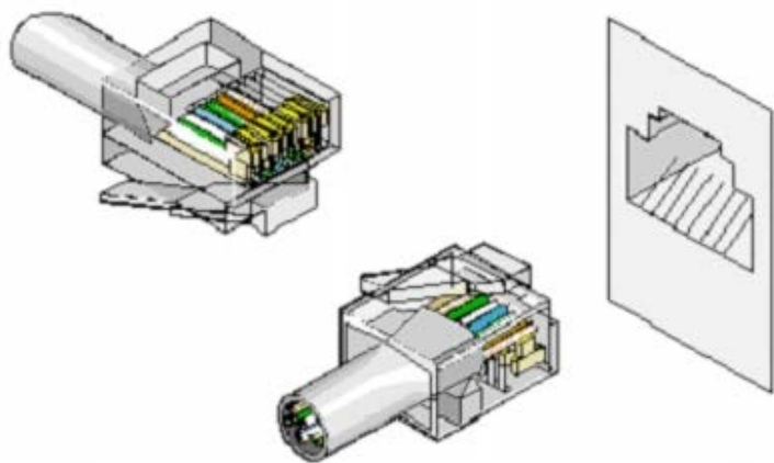
图 4-1. RJ-45 连接器
