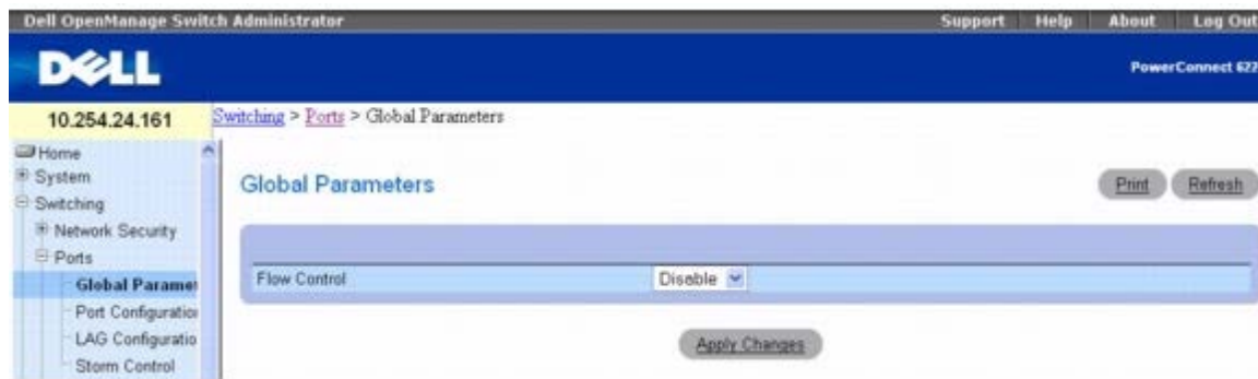
图 8-19. 全局参数
