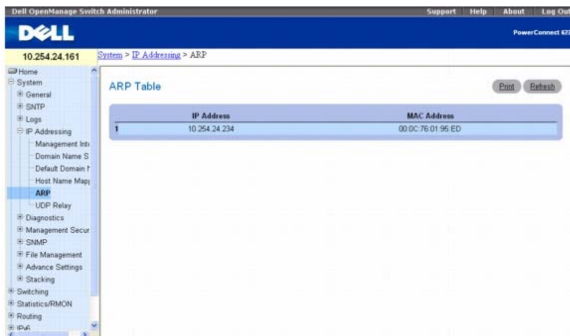
图 6-29. ARP 表
