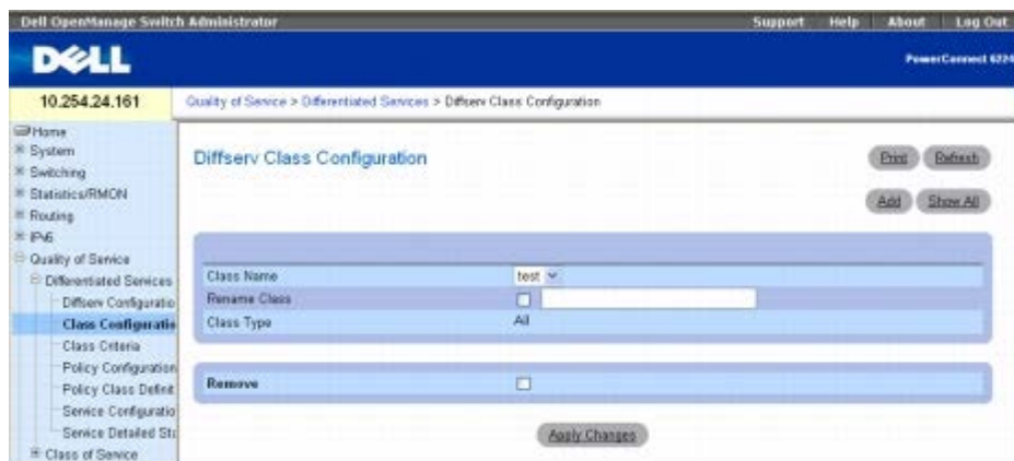
图 12-2. Diffserv 类配置
