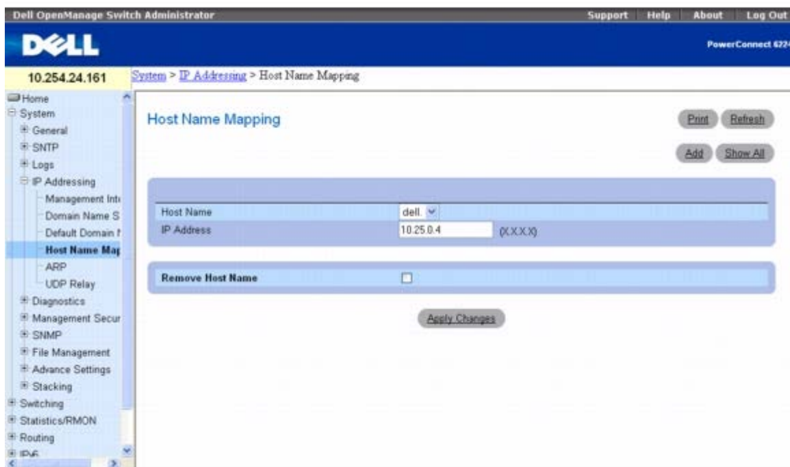
图 6-26. 主机名映射
