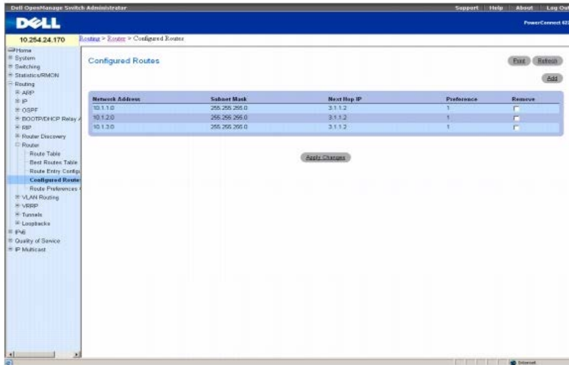
图 10-35. 配置的路由
