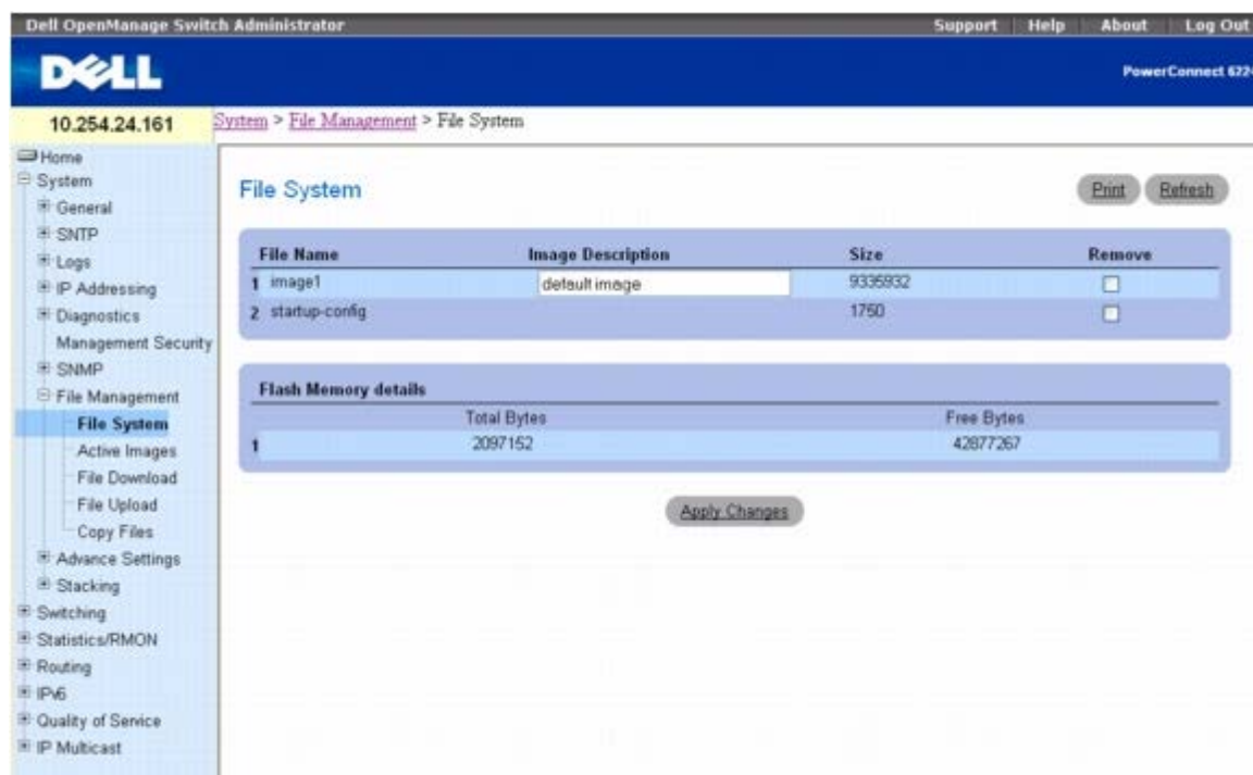
图 6-78. 文件系统
