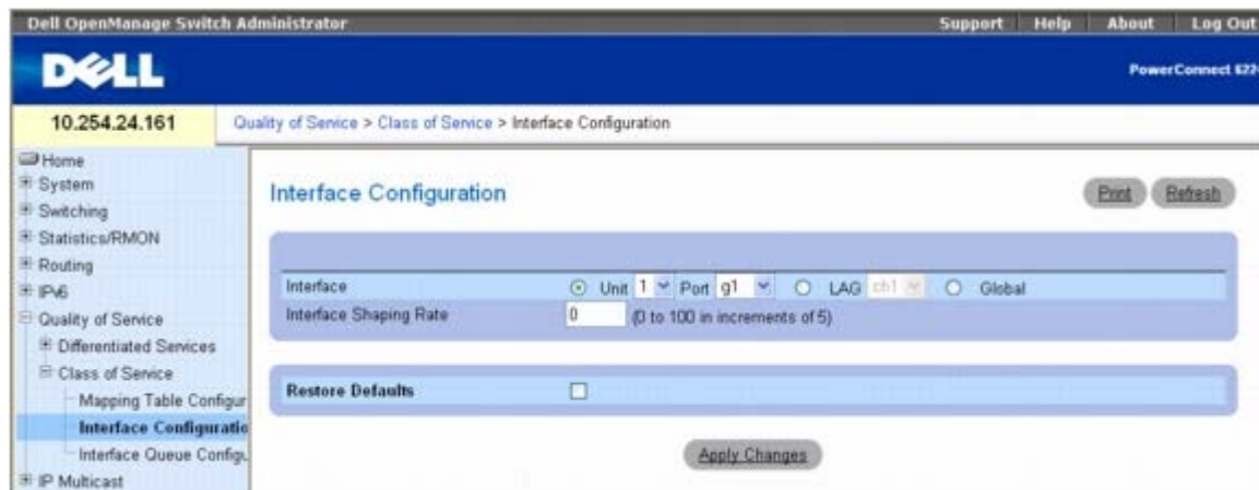
图 12-18. 接口配置
