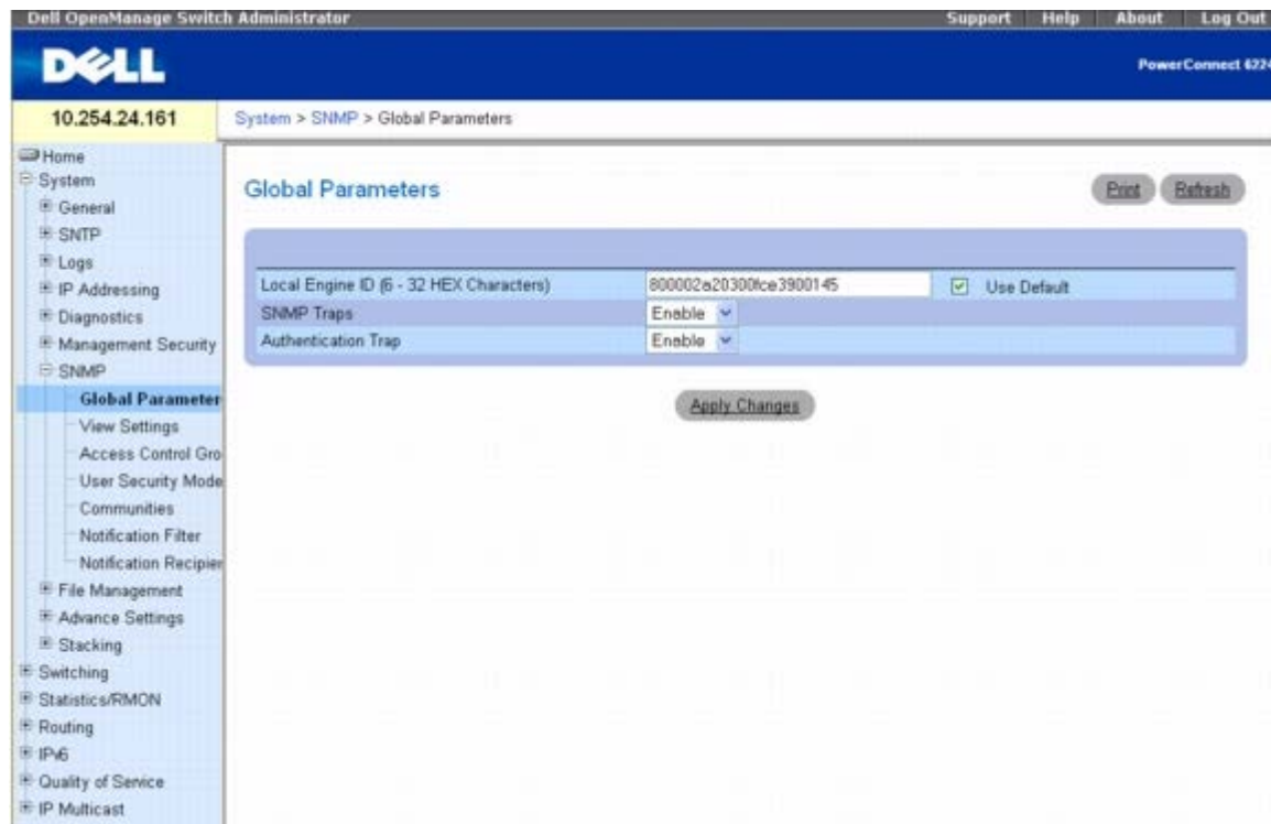
图 6-58. 全局参数
