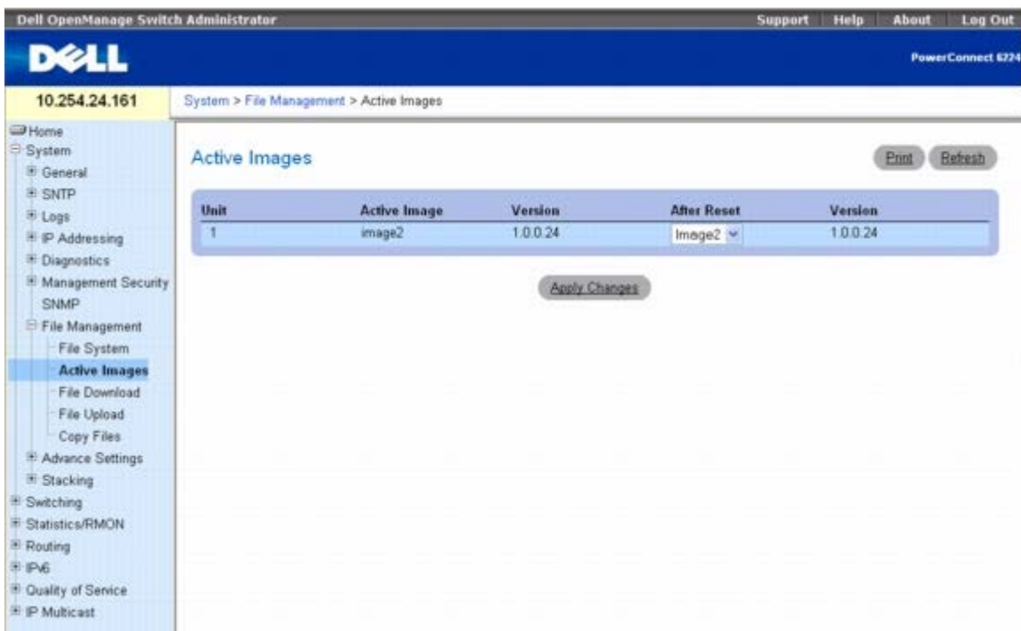
图 6-79. 活动映像
