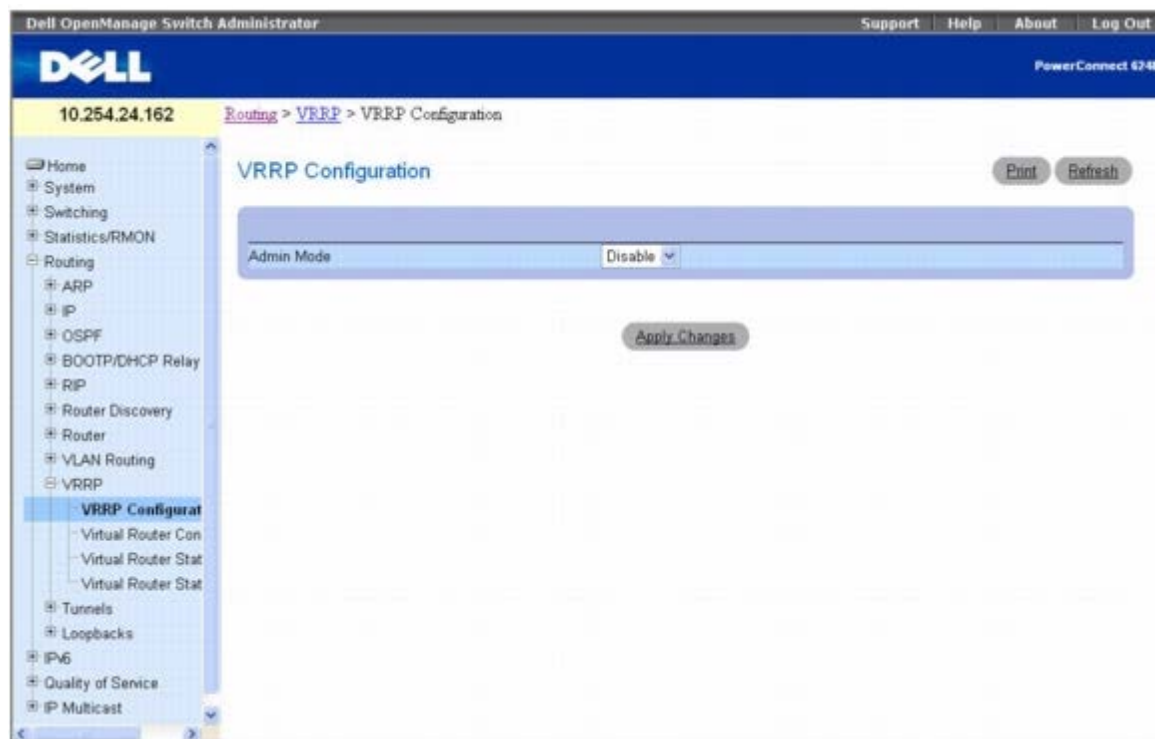
图 10-38. VRRP 配置
