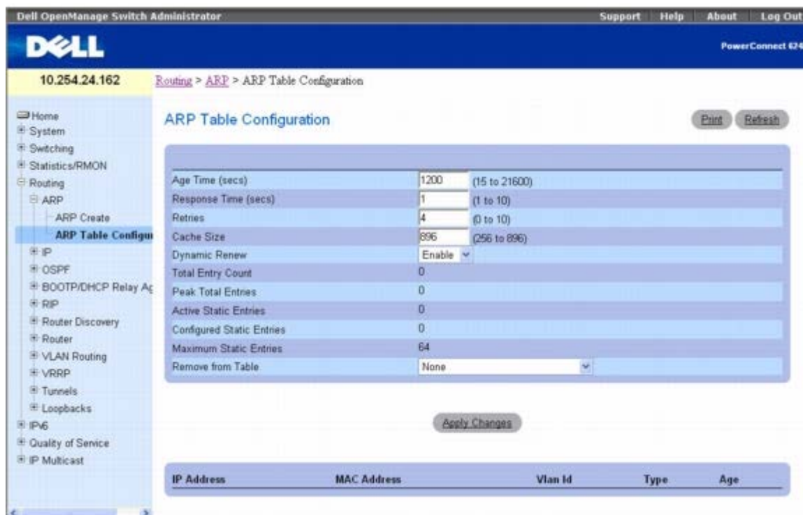
图 10-2. ARP 表配置
